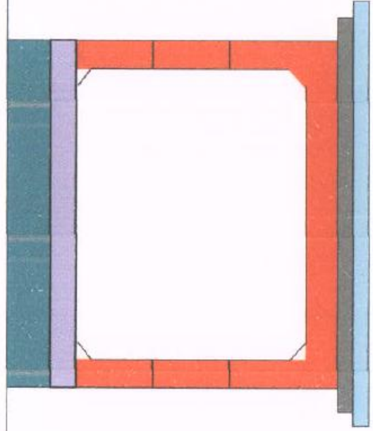
BOX CULVERT 16+600
